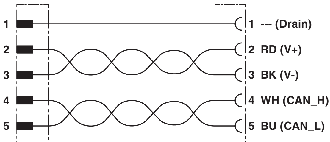
Diagrama eléctrico
