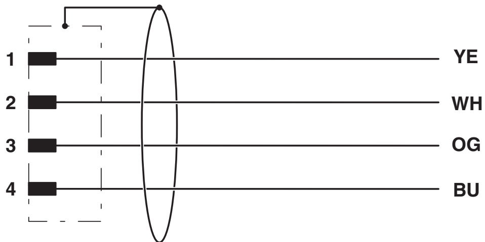
Schaltplan
