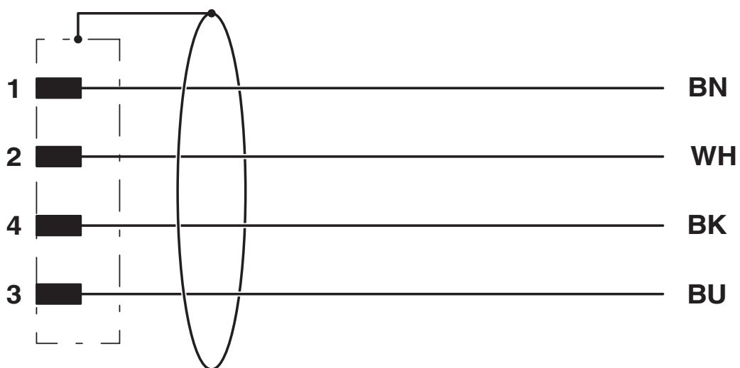
Kontaktbelegung der M12-Stecker
