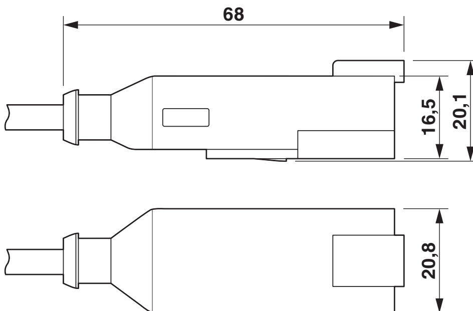
Dessin coté
