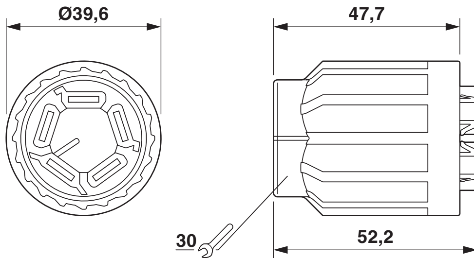
Dibujo acotado de la tuerca QPD 5 x 6,0
