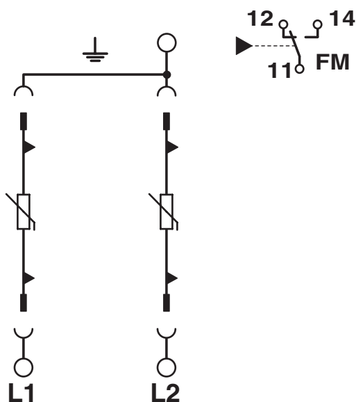
Diagrama eléctrico
