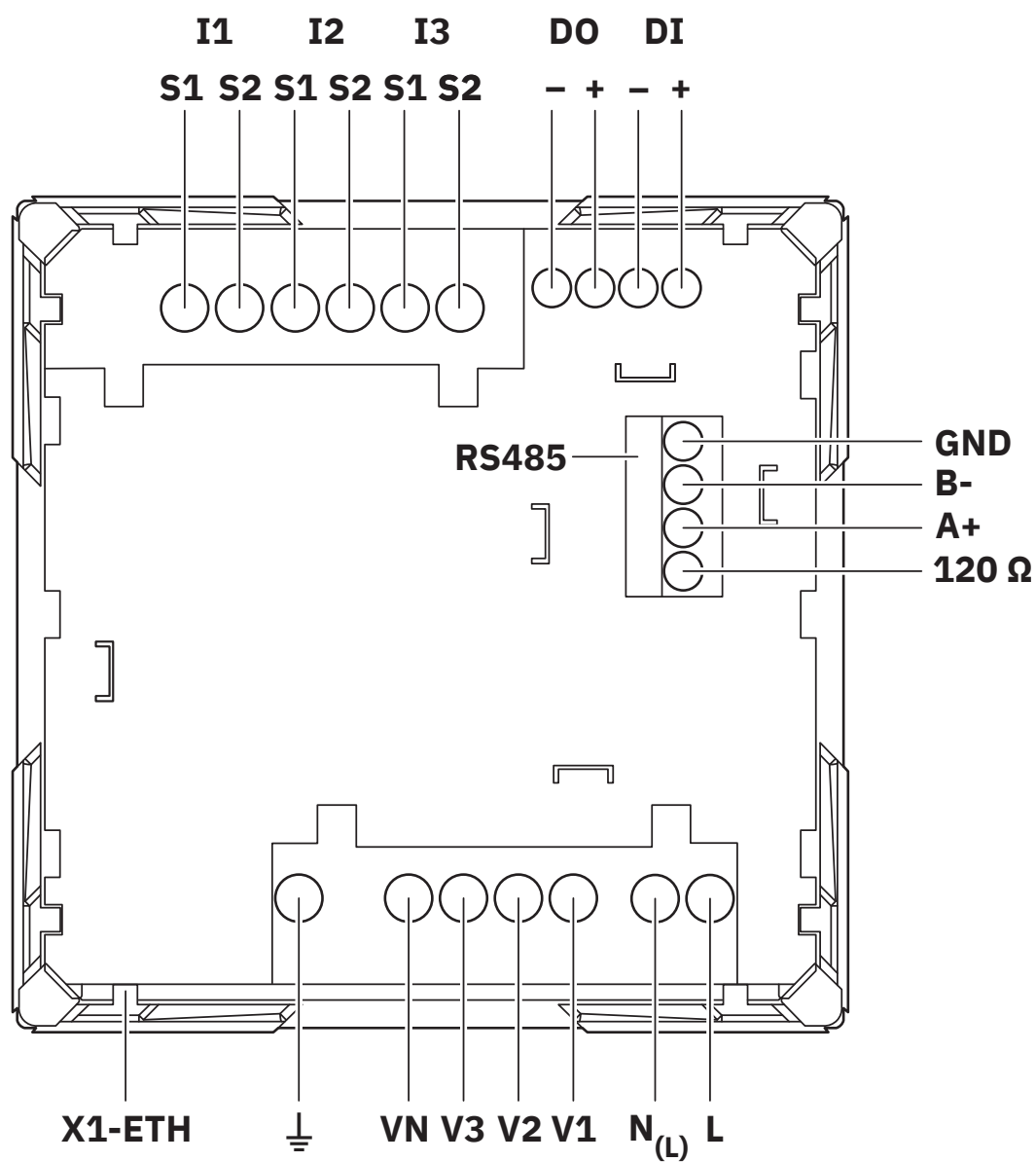
Dibujo de conexión
