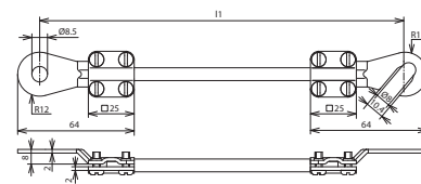
Maßbild EL10 L0.45M 1KSO 8.10 1KSG 8
