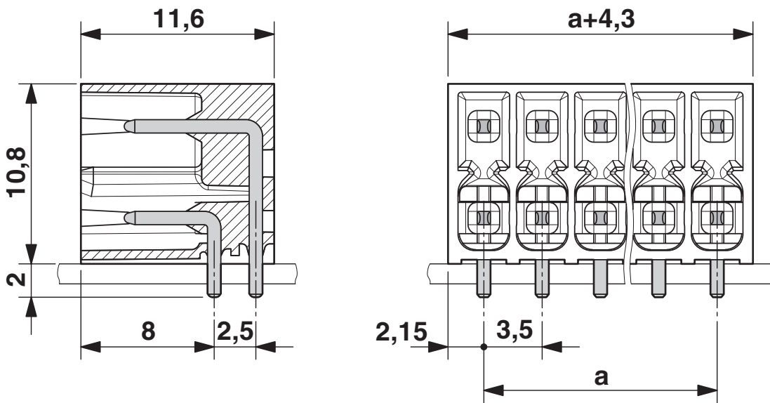
Dessin schématique
