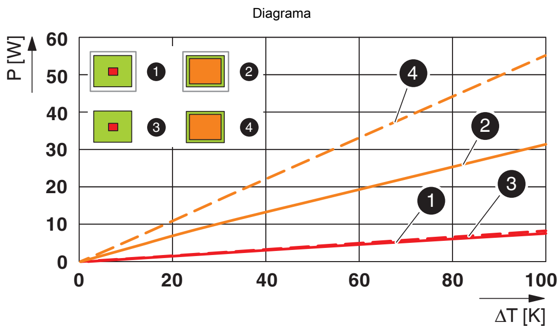
Diagrama de disipación de energía 0 K ... 100 K
