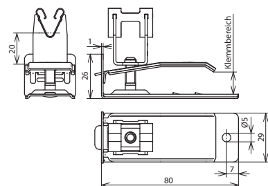
Maßbild DLH DG H20 UK8 V2A
