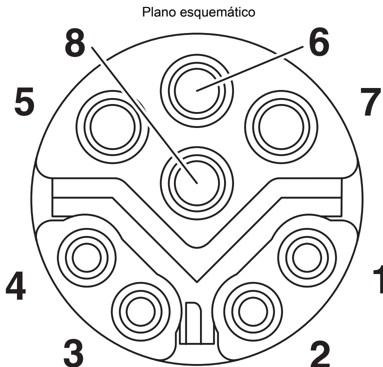
Esquema de polos conector híbrido M12, 8 polos, con codificación Y, vista lado hembra
