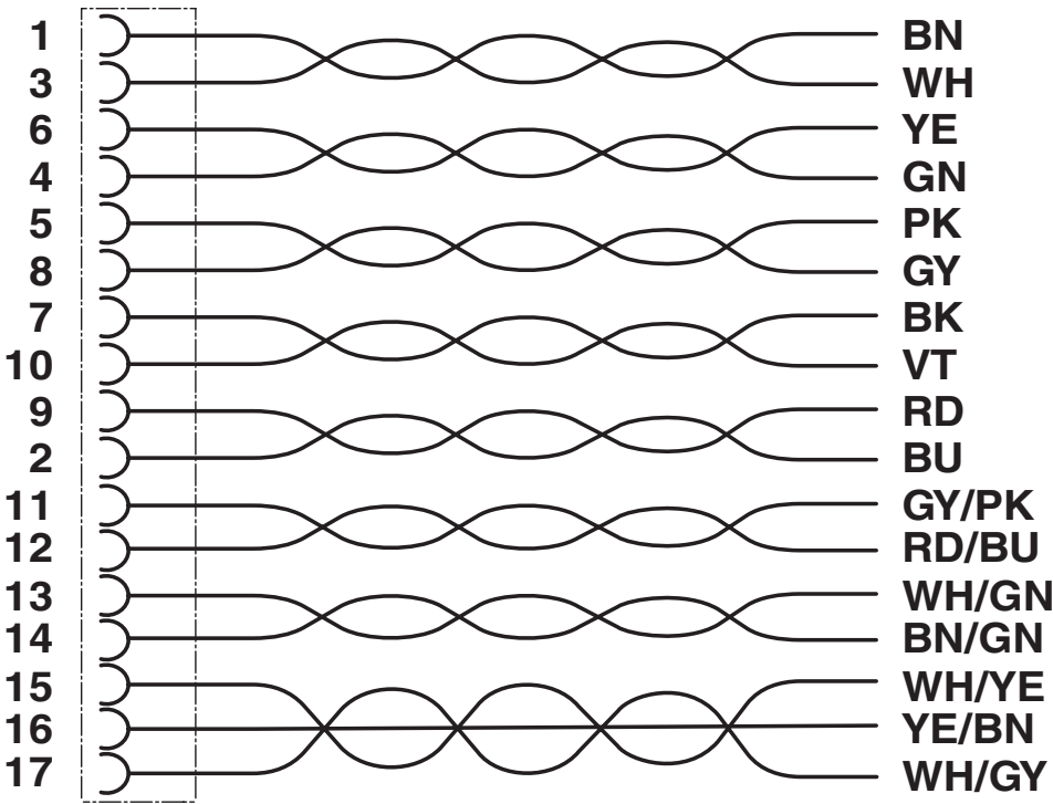
Diagrama eléctrico
