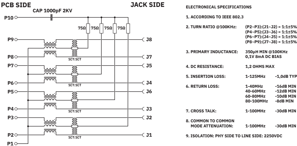
Diagrama eléctrico
