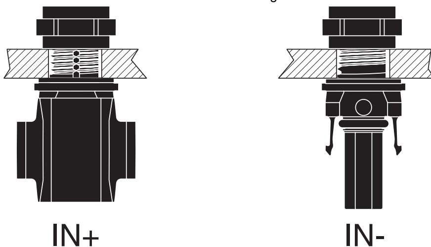
Schemazeichnung
