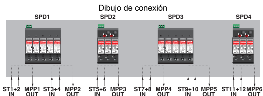
Plano esquemático
