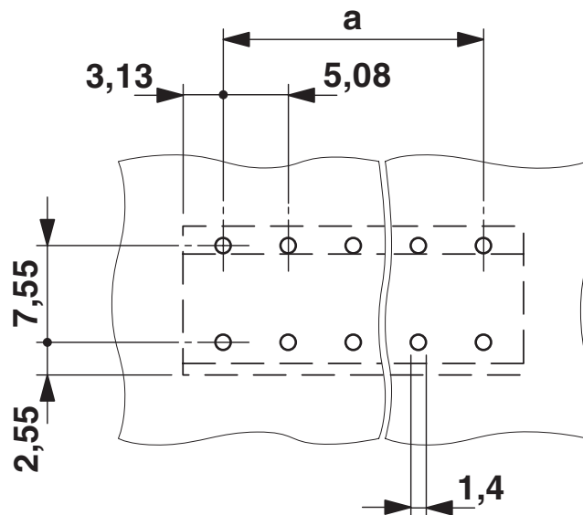
Bohrplan/Lötpadgeometrie
