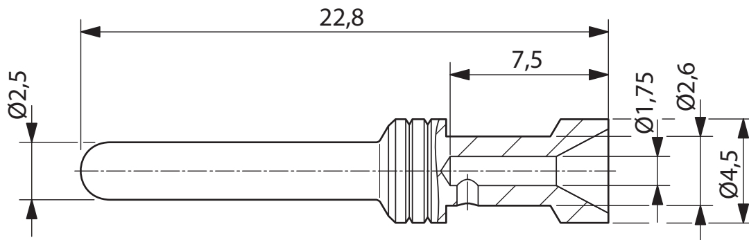
Dessin coté
