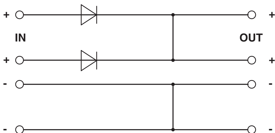
Schéma fonctionnel
