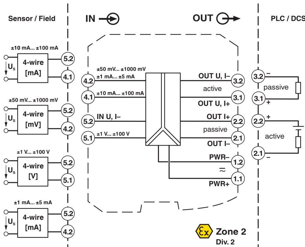
Schéma fonctionnel
