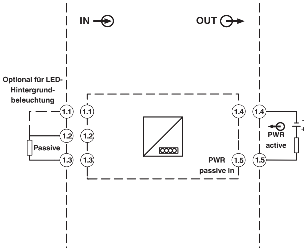
Blockschaltbild FA MCR-DS-I-I-OLP
