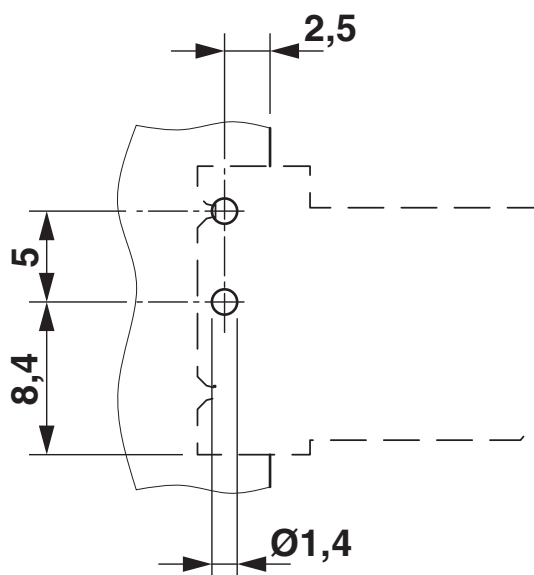
Bohrplan/Lötpadgeometrie
