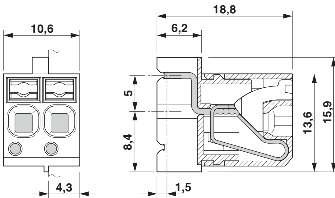
Maßzeichnung
