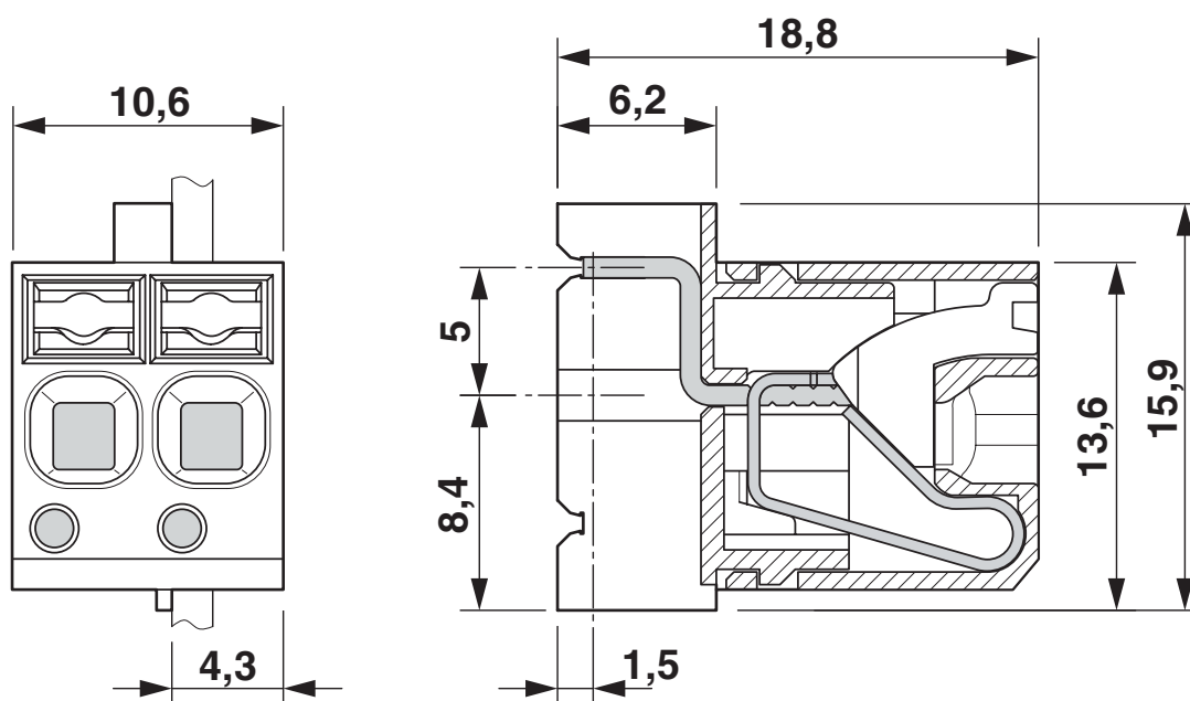
Dessin coté
