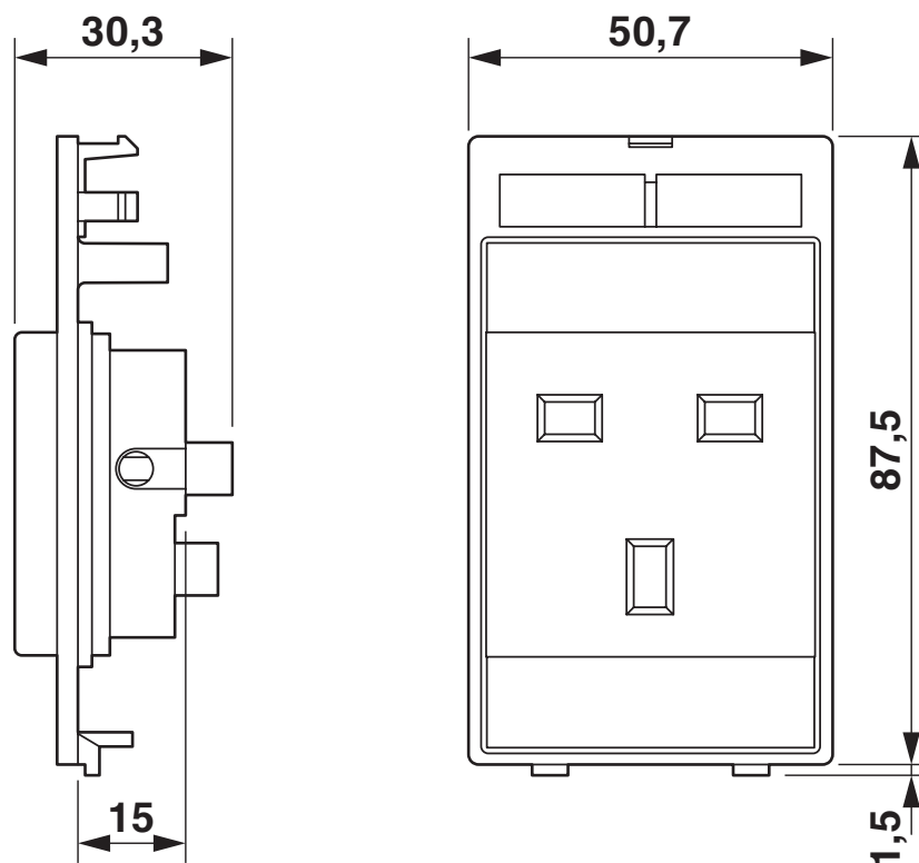
Dessin coté
