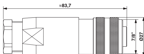
Esquema de dimensiones
