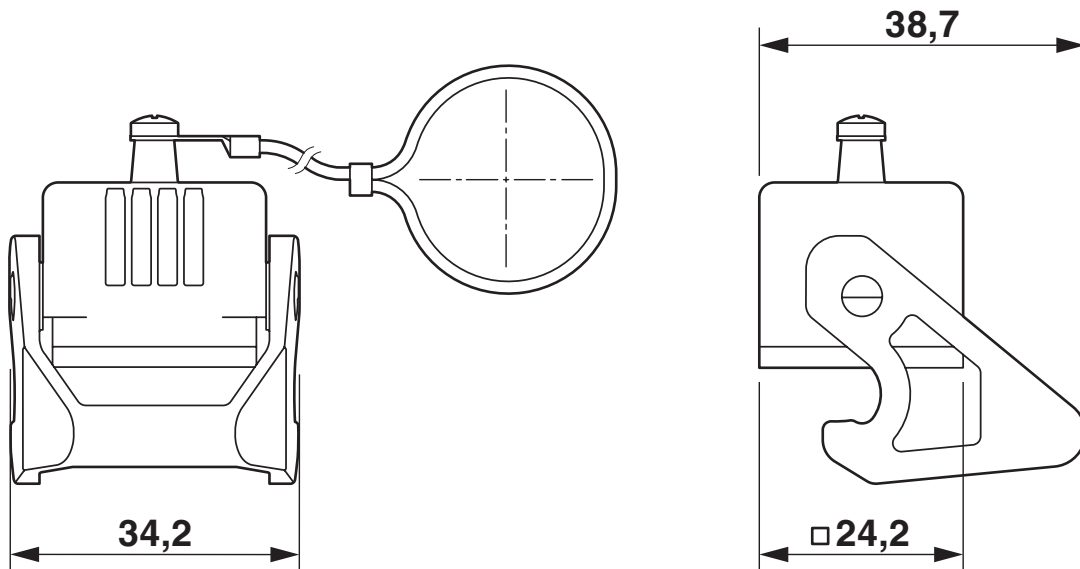
Maßzeichnung
