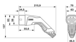
Fahrzeug-Ladestecker
