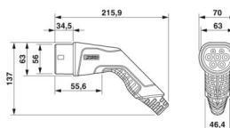
Connecteur de charge du véhicule
