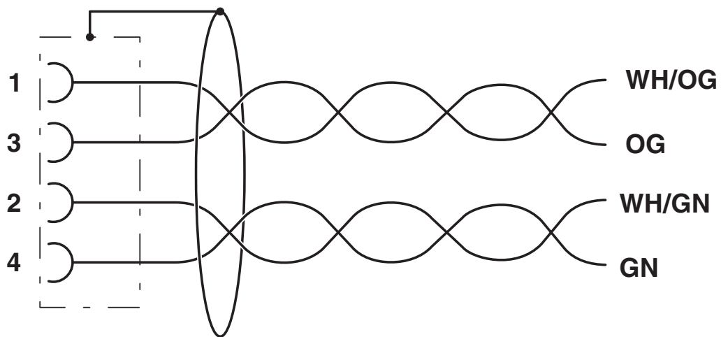
Schaltplan
