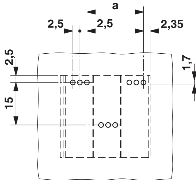
Bohrplan/Lötpadgeometrie
