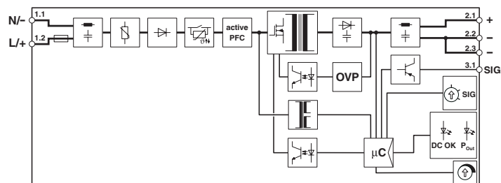
Blockschaltbild
