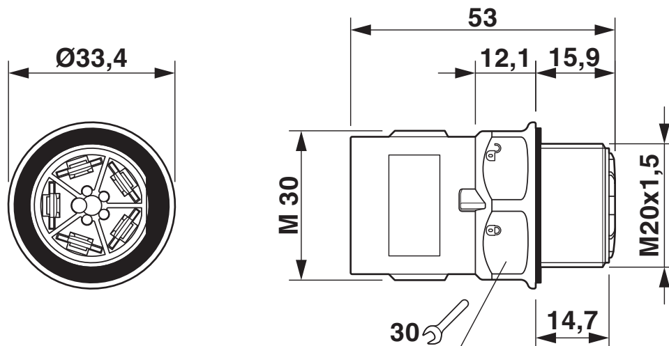
Maßzeichnung des QPD W 5x2,5 M20 ohne Mutter
