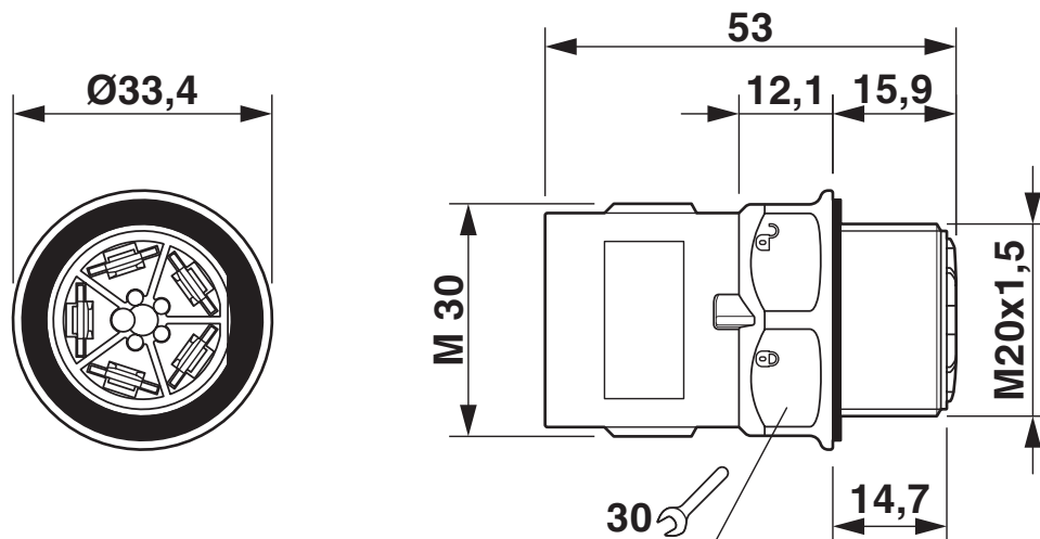
Dibujo acotado de QPD W 5 x 2,5 M20 sin tuerca
