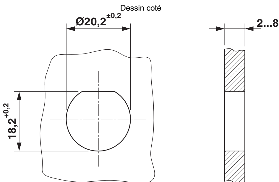
Dessin coté QPD W 5x2,5 M20 sans écrou
