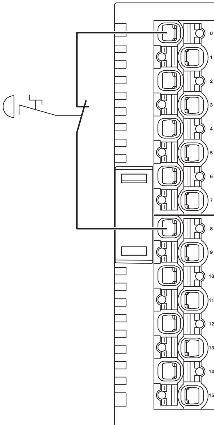
Conexión típica de un circuito de parada de emergencia
