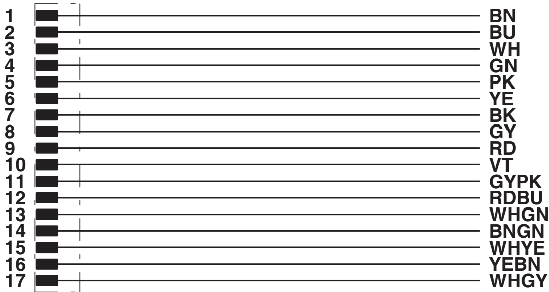
Ocupación de contactos del conector macho M12
