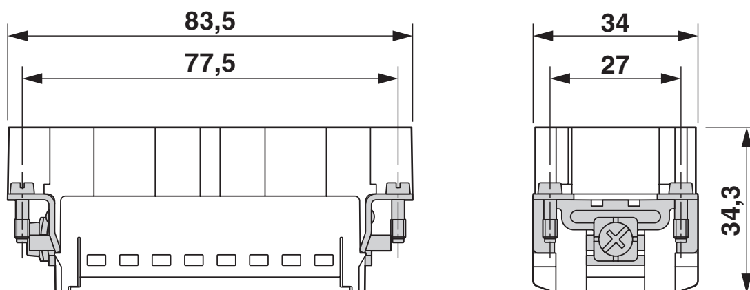
Dessin coté
