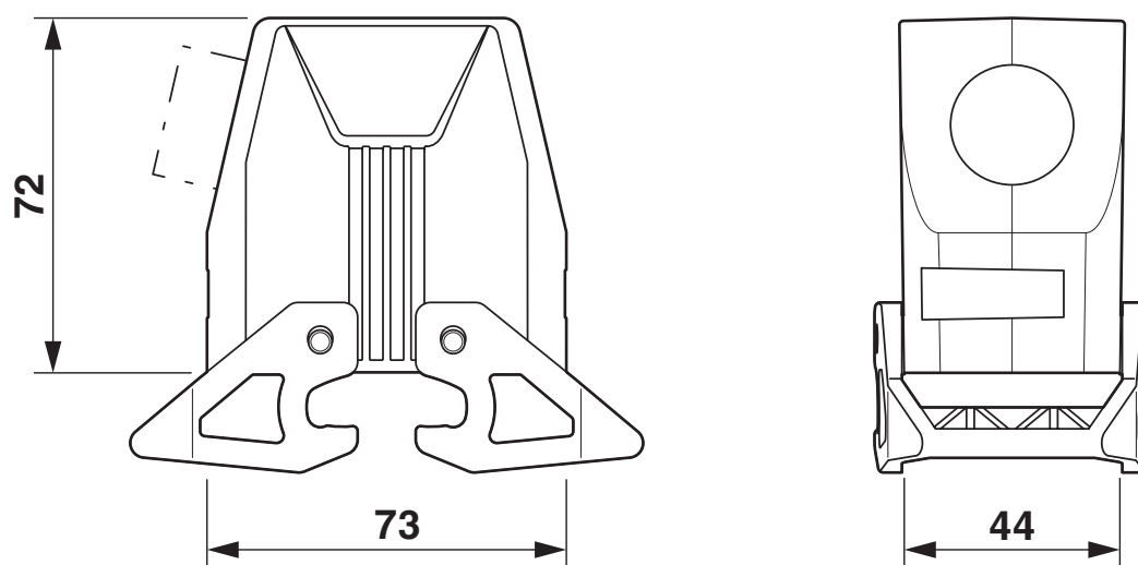
Dessin coté
