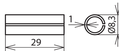
Maßbild CUPAH GL Q25 L29 AL CU
