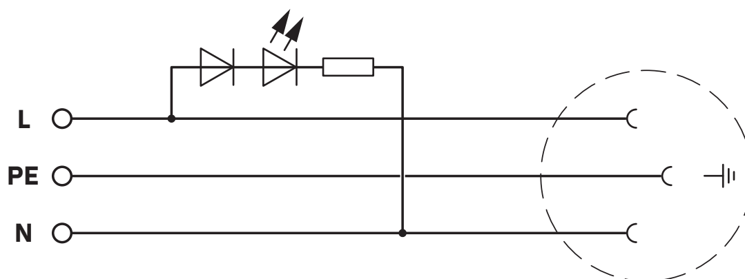
Diagrama eléctrico
