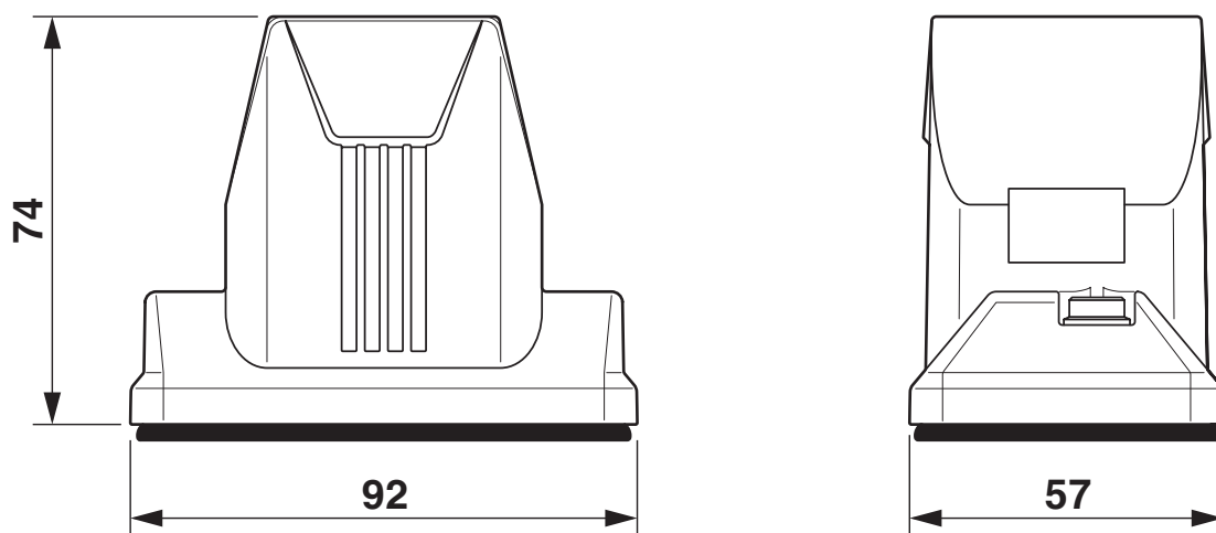
Dessin coté
