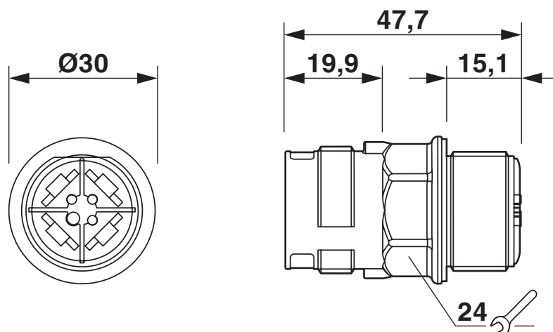
Dessin coté
