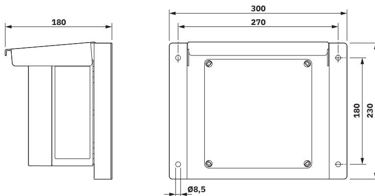
Dessin coté
