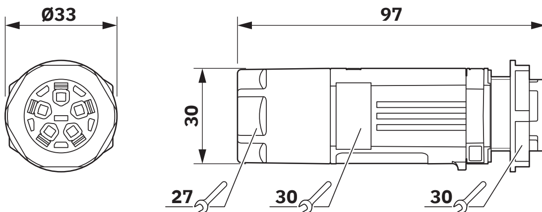
Maßzeichnung
