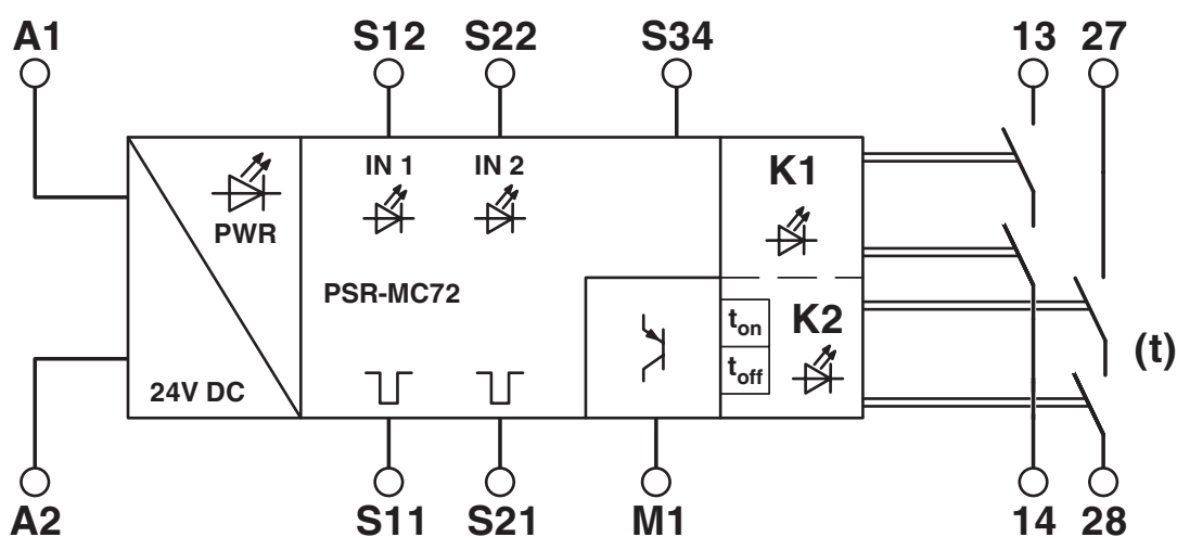
Schéma fonctionnel
