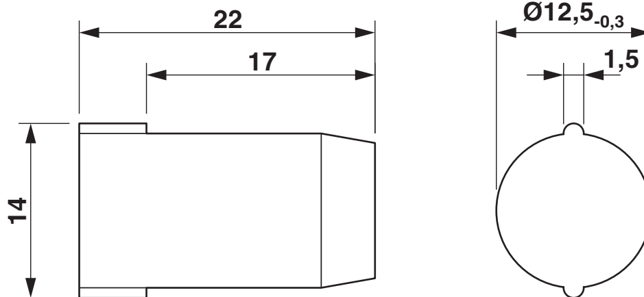
Maßzeichnung
