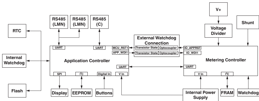
Schéma fonctionnel
