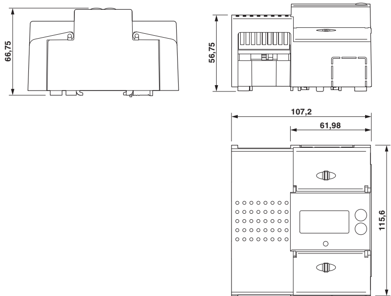
Dessin coté
