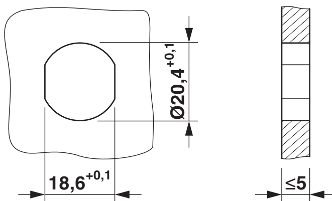
Gehäuseausschnitt für M20-Befestigungsgewinde, Montagewand mit Gewinde
