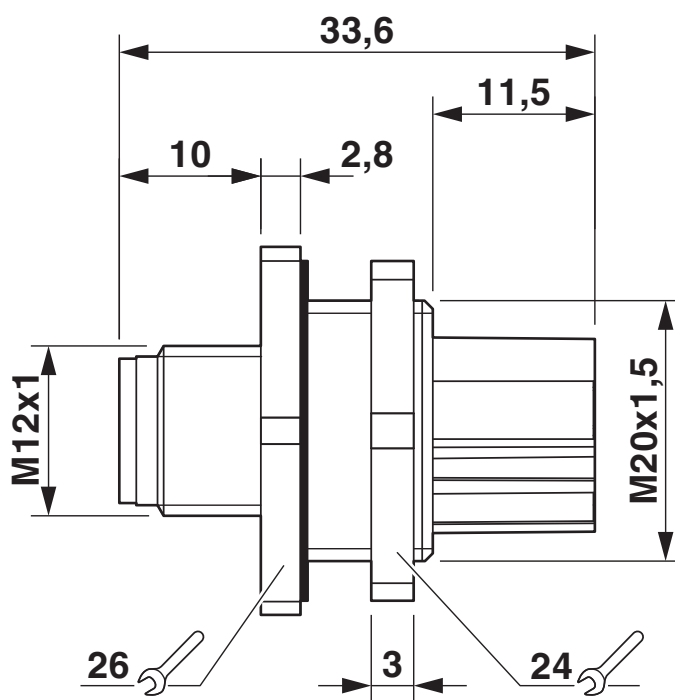
Maßzeichnung
