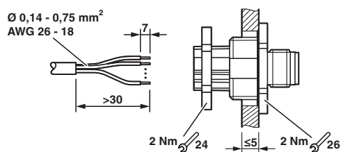
Funktionszeichnung
