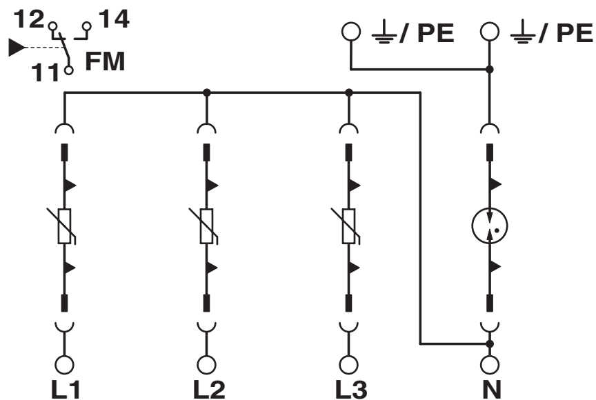
Schaltplan
