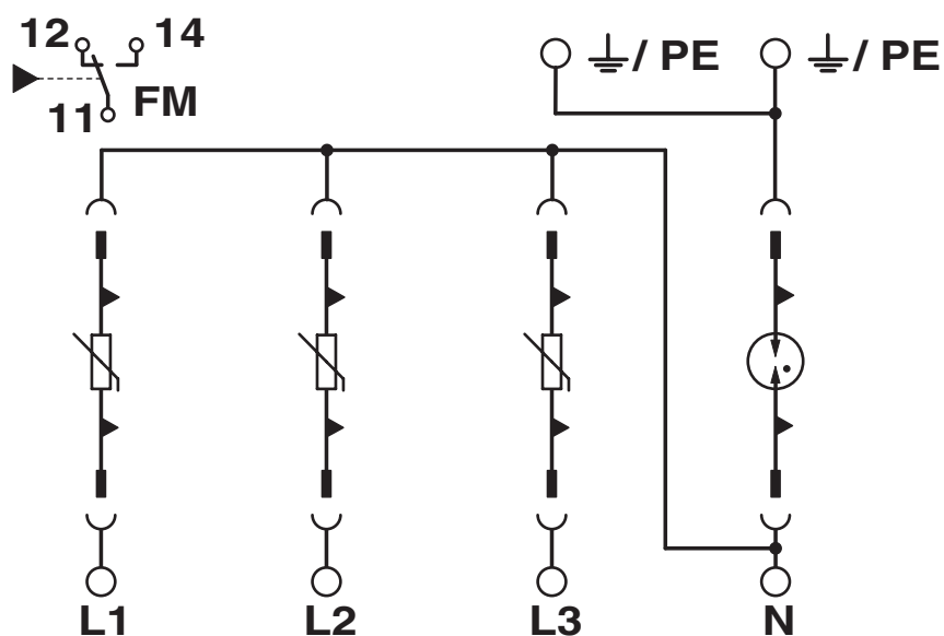
Diagrama eléctrico
